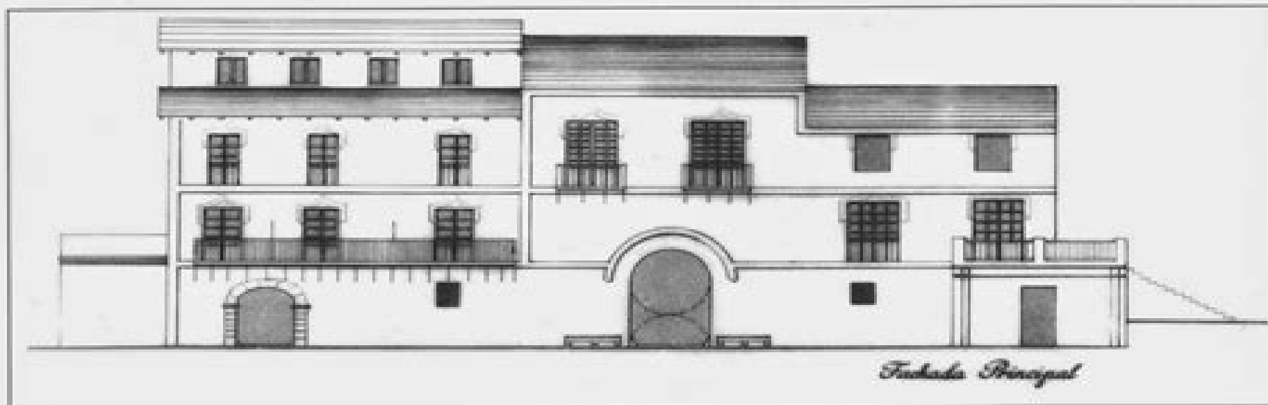
Casa El Pelegrí. Piso 1º: 1. Cup. 2. Bodega. 3. Vestíbulo. 4. Hogar de la cocina. 5. Dormitorio colono. 6. Cocina. 7. Pozo. 8. Vestíbulo. 9. Bodega. 10. Cub. Fachada Principal.
