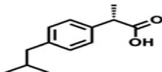
(S)-(+)-Ibuprofen
