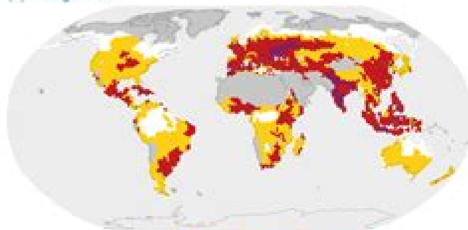
(d) Drought risk
