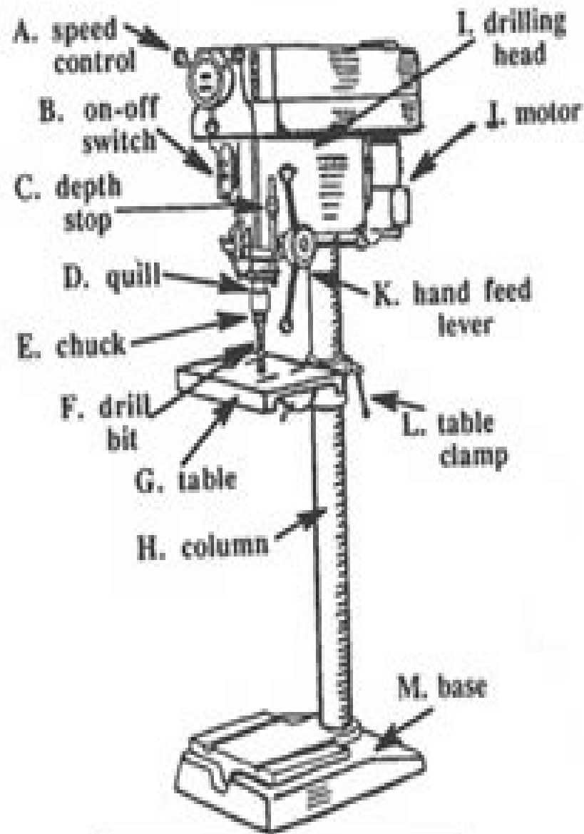
N. Sensitive Drill Press
