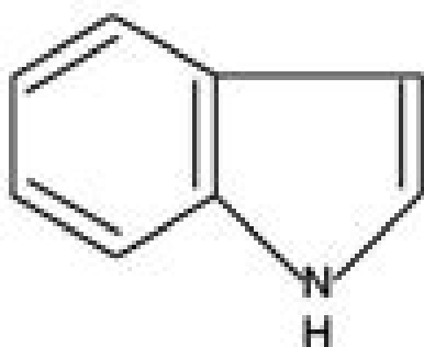
Indol
