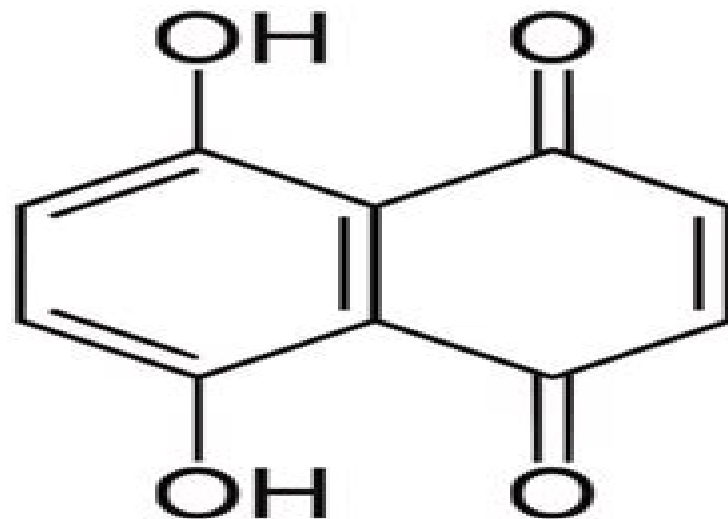
Naphthazarin
