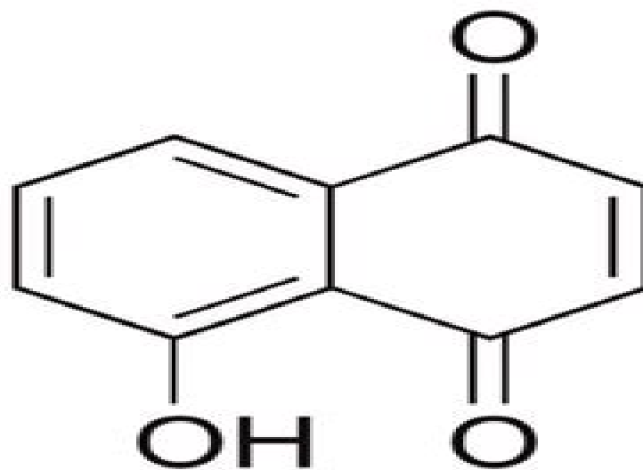
Lawsone
