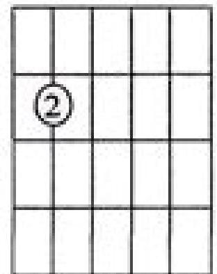
E minor7
