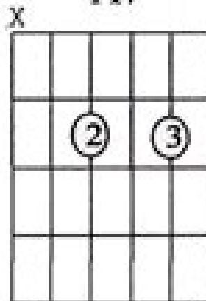
A7
