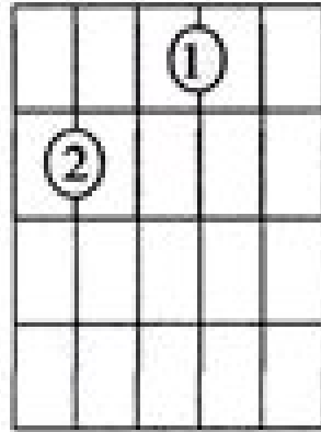
E7
